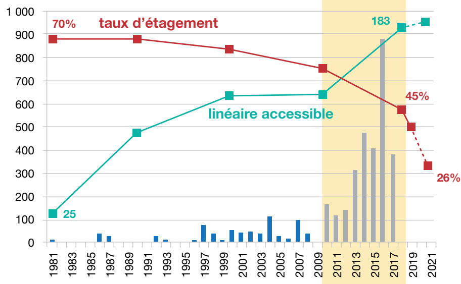
Figure 3. Restauration de la continuité écologique et réponse des effectifs de saumon dans le bassin de l'Orne. PARCE : Plan d'actions national pour la restauration de la continuité écologique des cours d'eau. (Source : Agence de l'eau Seine Normandie).
