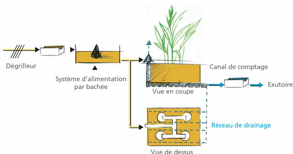
Figure 4. Schéma de la filière tropicale.
