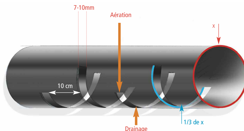
Figure 22. Schéma des canalisations d'aération-drainage.
