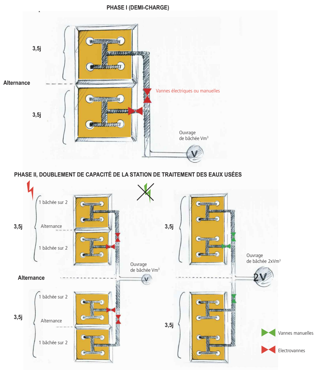
Figure 18. Phasage d'un projet de filtre planté de végétaux (FPV) par partitionnement ou ajout d'une nouvelle file eau.
